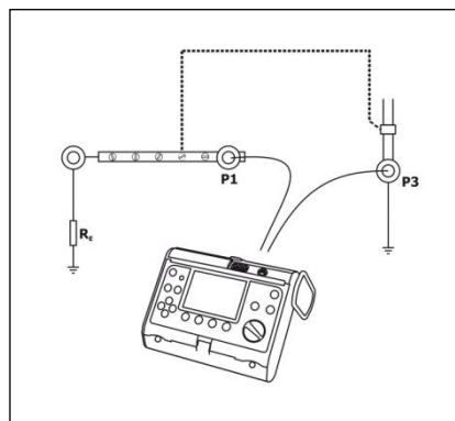
Рис 17. Подключение измерителя.
