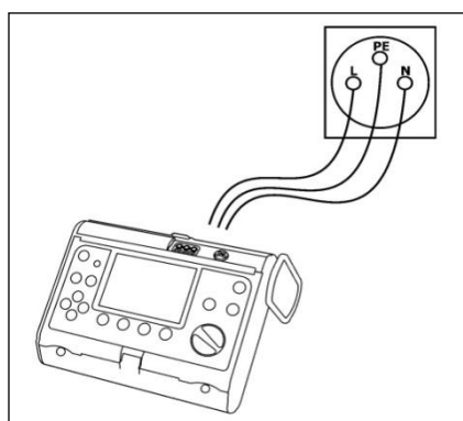
Рис.6. Подключение прибора.
