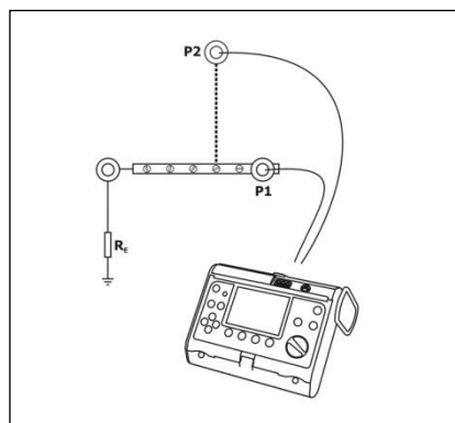
Рис. 16. Подключение прибора.
