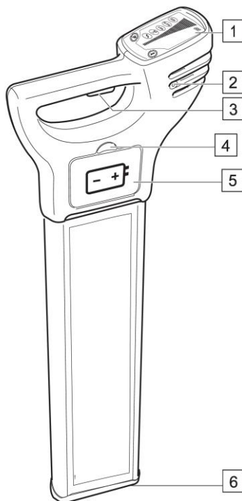
Описание конструкции приёмника LKO-1000
