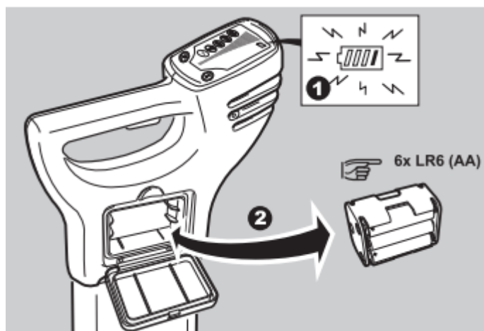
Замена элементов питания в приёмнике LKO-1000
