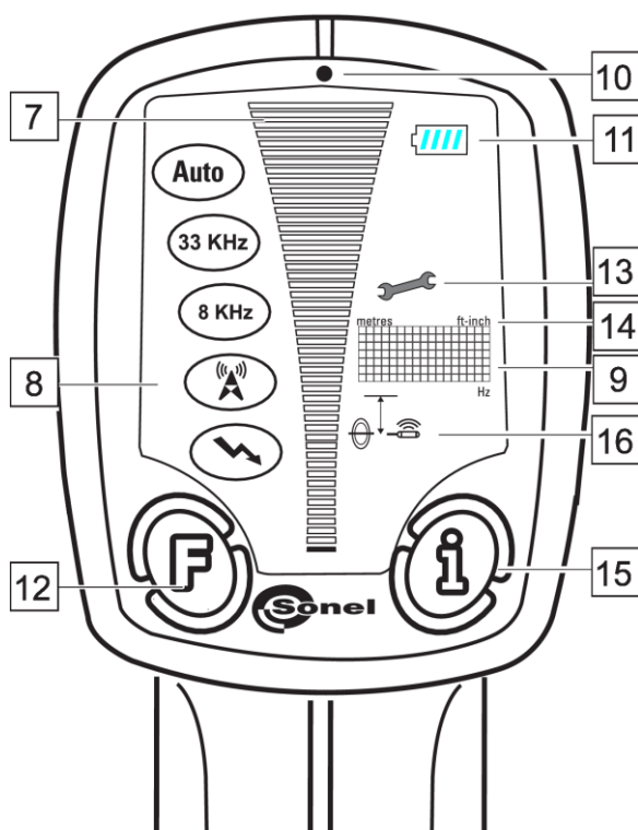
Панель индикатора приёмника LKO-1000
