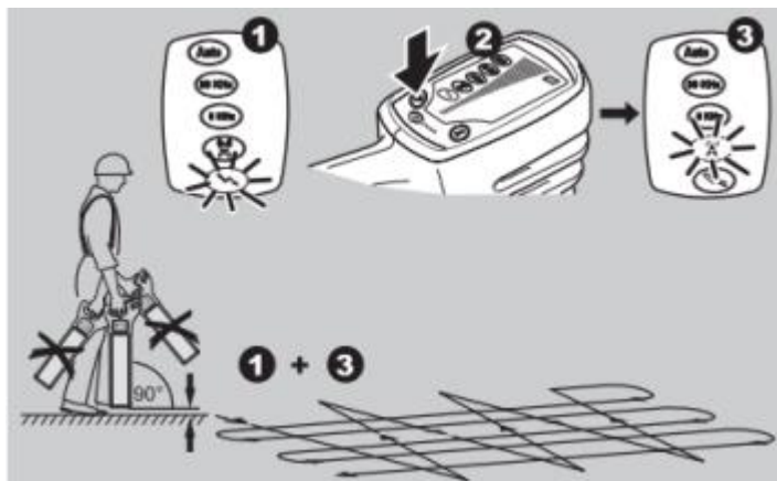
Непрерывный поиск/сканирование в режимах Power и Radio
