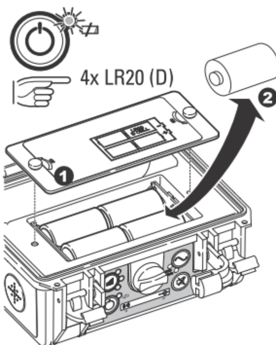
Замена элементов питания в генераторе LKN-1000
