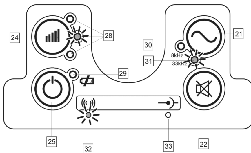
Лицевая панель генератора LKN-1000
