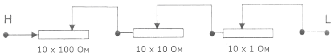
Рис.1. Схема соединения декад резисторов на примере магазина MC-3-Y-100-1
