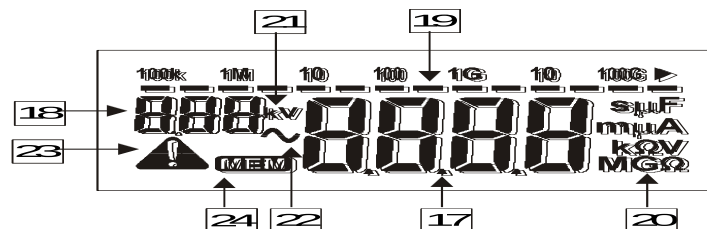
Рис.2. Жидкокристаллический дисплей
