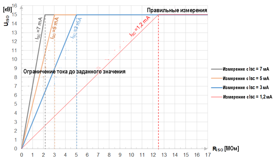
Фактическое напряжение измерения U_{iso} в функции измерения сопротивления изоляции R_{iso} (для максимального измерительного напряжения)
