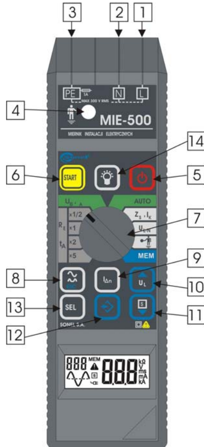
Рис.1. Расположение гнезд и клавиш в приборе MIE-500 (лицевая панель)
