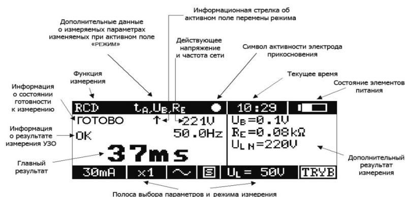
Рис.2. Отображение информации на дисплее
