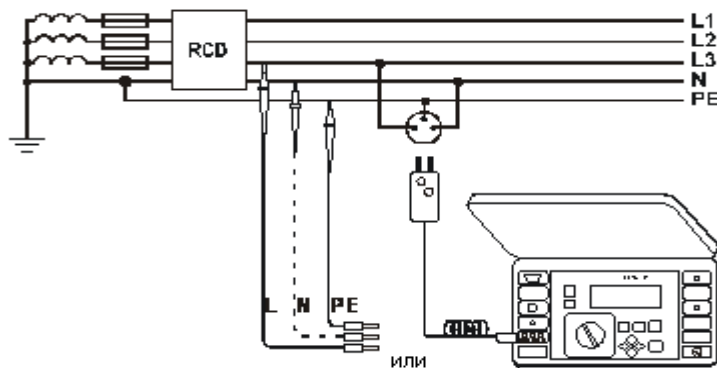
Рис.16. Измерение в цепи, оснащенной УЗО, при помощи зондов с острием или при помощи зонда в виде вилки (нулевой провод нужен только для тока ( I_{\Delta n} ) постоянного и пульсирующего, его отсутствие сигнализируется сообщением на дисплее.
