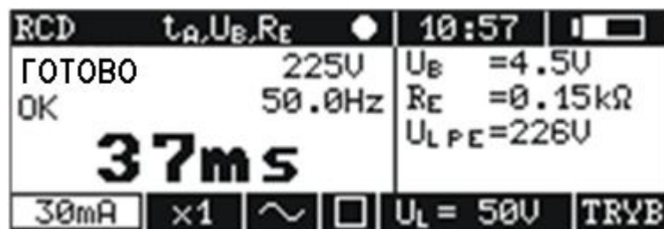
Рис.20. Отображение информации на дисплее при измерении времени отключения УЗО
