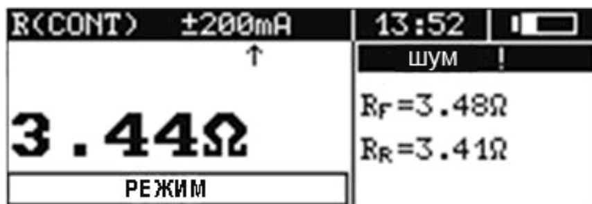
Рис.33. Отображение информации на дисплее при измерении целостности соединения током \pm 200 мА
