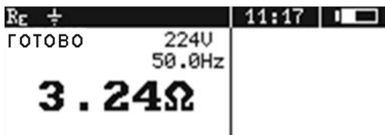
Рис.15. Отображение информации на дисплее при измерении сопротивления заземления
