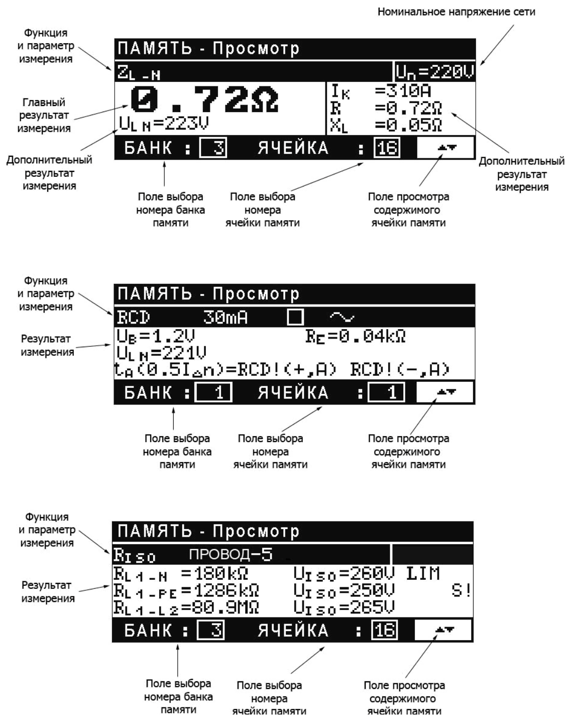
Рис.4. Отображение информации на дисплее при просмотре памяти :
