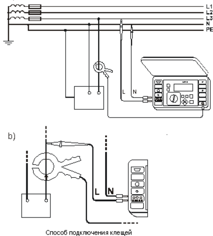
Рис.42. Схема измерения для сбора данных и измерения тока, мощности и \cos\varphi
