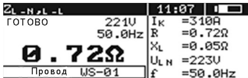
Рис.9. Отображение информации на дисплее при измерении параметров петли короткого замыкания
