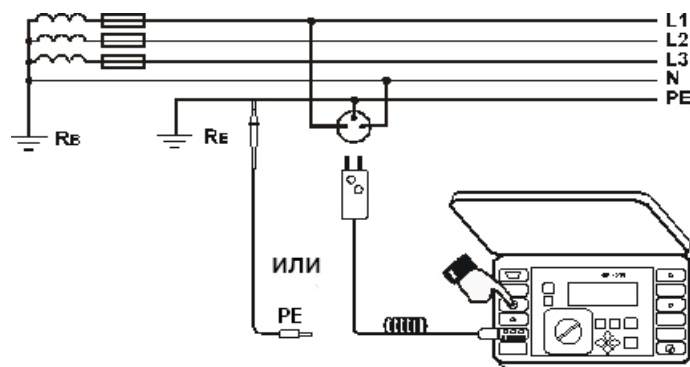
Рис. 6. Проверка правильности подключения защитного провода
