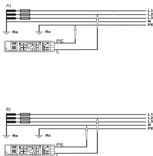
Рис. 8. Подсоединение прибора к электрической сети для измерения параметров цепи короткого замыкания: А) измерения между линиями L и PE, В) измерения между линиями L и N (провод N сети должен быть подсоединен к измерительному гнезду PE прибора)
