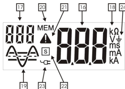
Рис.2 Дисплей на жидких кристаллах
