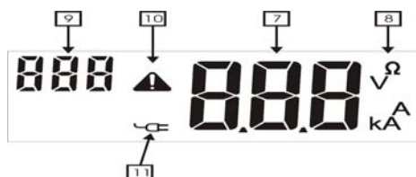
Рис.2. Дисплей измерителей семейства MZC-200
