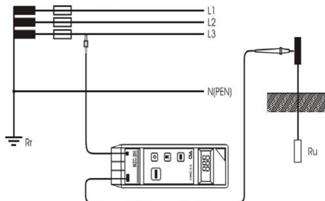
Рис. 10. Способ подключения измерителя семейства MZC-200 при измерениях сопротивления заземления
