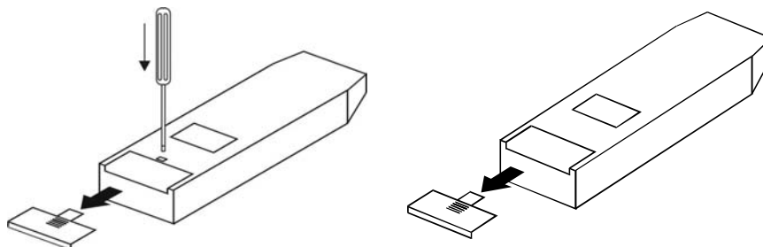
Рис.4. Вскрытие отсека элементов питания в приборах семейства MZC-200
