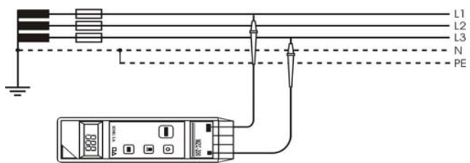
Рис.7. Измерение в рабочей цепи (L-L)
