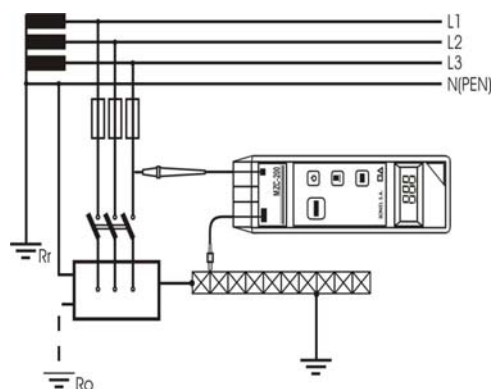
Рис. 11. Контроль целостности нулевых защитных проводников и уравнивательных соединений.
