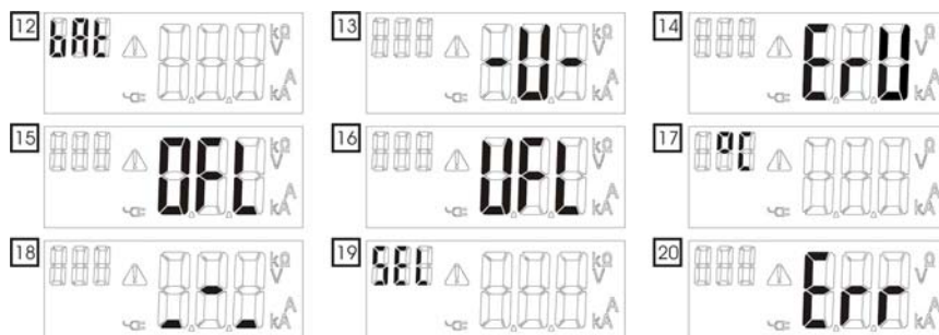
Рис. 3. Надписи и символы, отображаемые на дисплее измерителей семейства MZC-200
