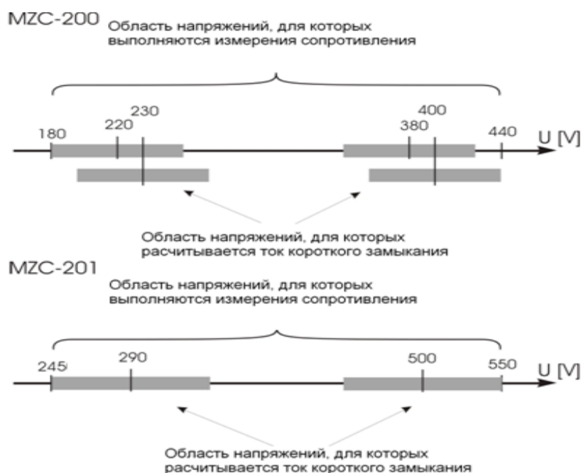
Рис. 9. Зависимости между напряжением сети и возможностью вычисления ожидаемого тока короткого замыкания на примере MZC-200 и MZC-201
