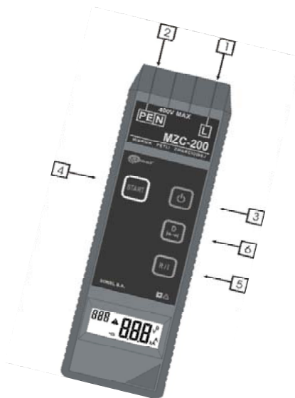
Рис.1. Расположение гнезд и клавиш в измерителях семейства MZC-200 (лицевая панель)
