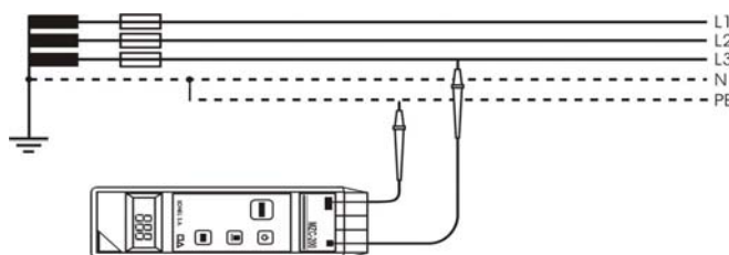
Рис.6. Измерение в защитной цепи (L-PE)
