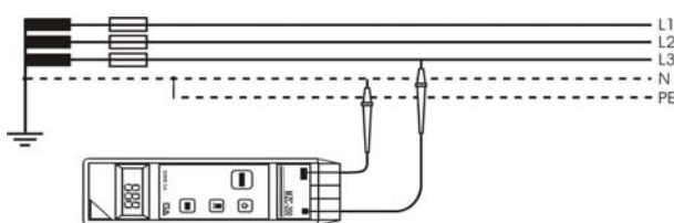
Рис.5. Измерение в рабочей цепи (L-N)
