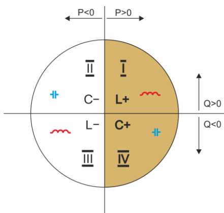
Рис.46. Четырехквадрантное деление потока мощности и энергии.
